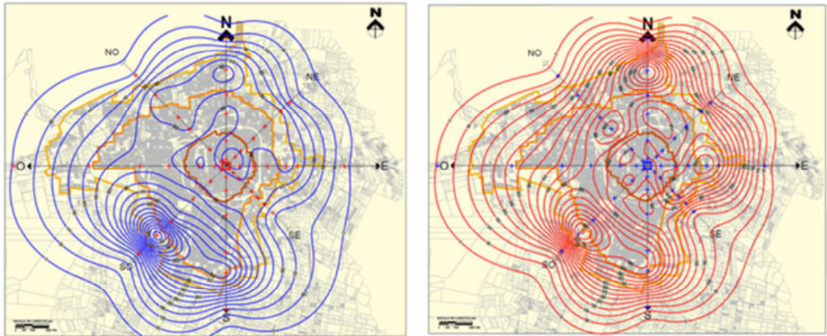
Fig. 2: Isolíneas de Energía Eléctrica y Gas por vivienda en el AMSJ – INVIERNO
