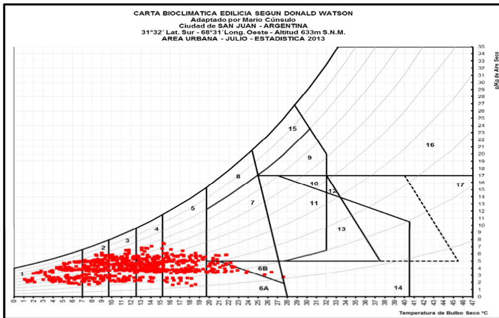
Fig. 5: Carta Bioclimática Edilicia AMSJ - Julio de 2013
