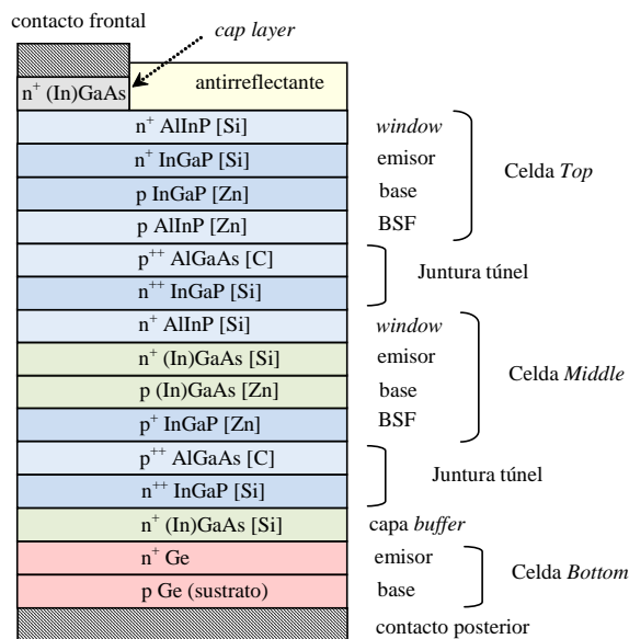
Fig. 7. Estructura de capas de una celda solar de triple juntura estándar. La capa 'cap layer' tiene como función proveer un buen contacto eléctrico en la interfaz metal-semiconductor. Fuente: Takamoto et al., 2000.
