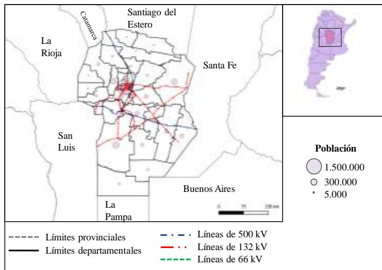
Fig. 1: Localización geográfica de la provincia de Córdoba. Población por departamento y líneas de alta tensión eléctrica.
