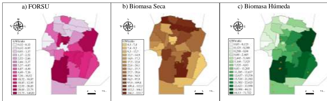
Fig. 3: Potencial energético técnico discriminado por tipo de biomasa a) FORSU, b) BS y c) BH. En b) y c) se georreferenciaron los 3 proyectos de biomasa (símbolo: hojas) y los 13 de biogás (símbolos: llamas) de las diferentes rondas del plan Renovar.
