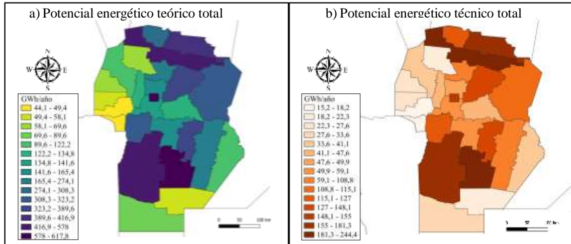
Fig. 2: Potencial energético a) teórico y b) técnico total, de acuerdo a la ecuación (4a y 4b).
