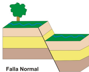
Falla Normal
