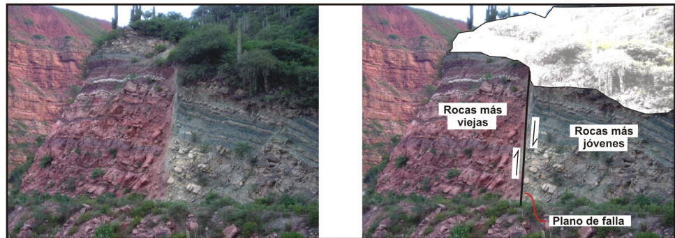
Falla Normal
