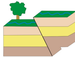
Falla Inversa
