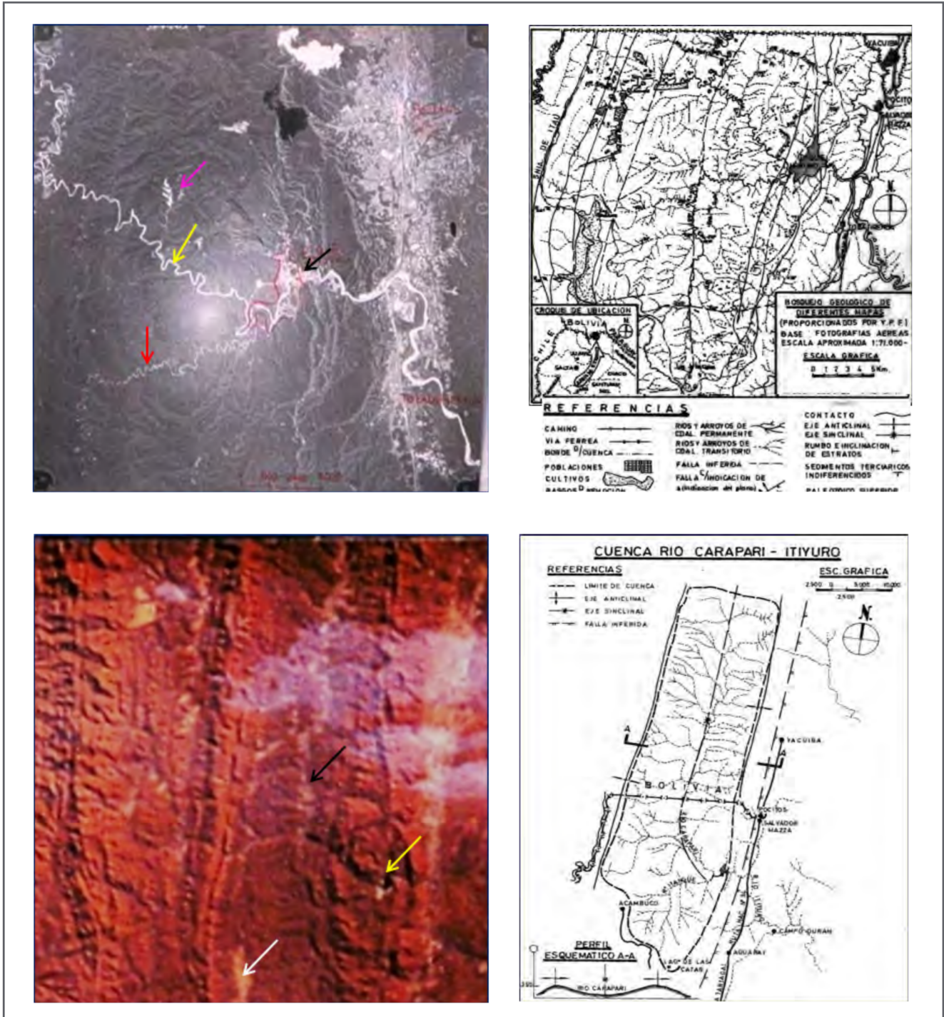
Figura 3. Arriba Izquierda: Fotografía aérea tomada por el IGM en 1966. Las flechas indican: la ubicación de la presa (negra), el río Carapari (amarilla), el río Itangüe (roja) y un área desestabilizada activa (magenta). Arriba Derecha: Mapa resultante de la interpretación de la totalidad de la cuenca en el territorio argentino. Abajo Izquierda: Imagen satelital bandas 4, 5 y 7 de fecha 27/07/81 de la cuenca total del dique. Las flechas indican: el espejo de agua (amarilla), el río Carapari en territorio boliviano (negra) y el paraje de Acambuco (blanca). Abajo Derecha: Mapa integrado de la cuenca completa desarrollada en ambos países.
