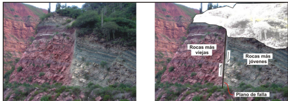
Falla Normal
