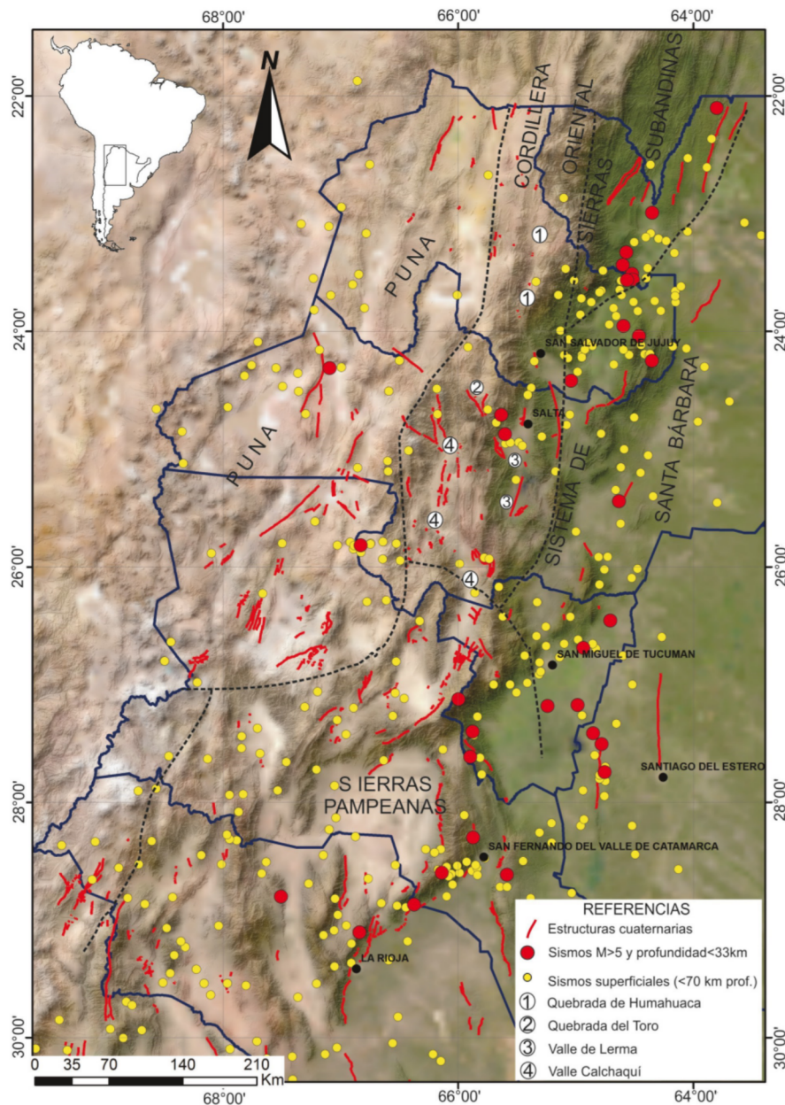
Mapa del NOA con principales estructuras cuaternarias, sismos someros y límite de provincias geológicas (Tomado de Casa A, Yamin M, Wright E, Costa C, Coppolecchia M, Cegarra M, y Hongn F (Eds.). 2014. Deformaciones Cuaternarias de la República Argentina, Sistema de Información Geográfica. Instituto de Geología y Recursos Minerales, Servicio Geológico Minero Argentino).
