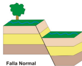
Falla Normal
