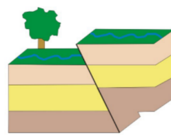
Falla Inversa
