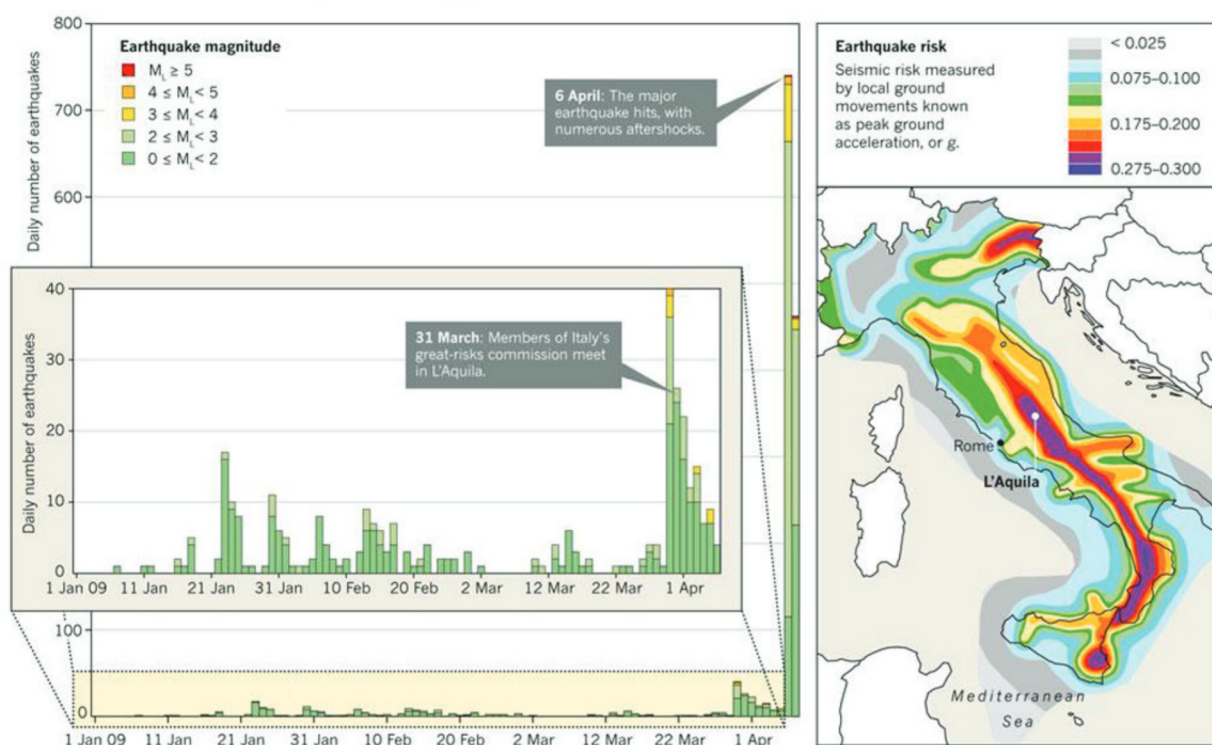
Figura 1. Mapa tomado de la revista Nature cuya fuente citada es el INGV. A la izquierda se muestra un gráfico con la cantidad de sismos registrados por día, con la barra de color indicando la magnitud. Los sismos son mostrados en detalle en el gráfico interno. Derecha: Mapa de peligrosidad sísmica de Italia.
