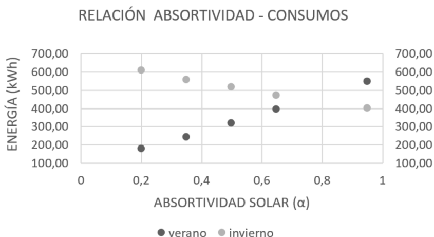
Fig. 5: Relación de la absortividad solar ( \alpha ) de la placa exterior y los consumos energéticos (kWh) para climatización en el estar
