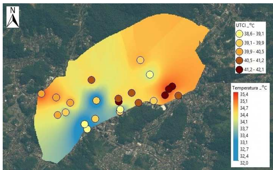
Figura 9: Mapa de temperatura do ar associado aos resultados para o índice de conforto UTCI – ArcGis.
