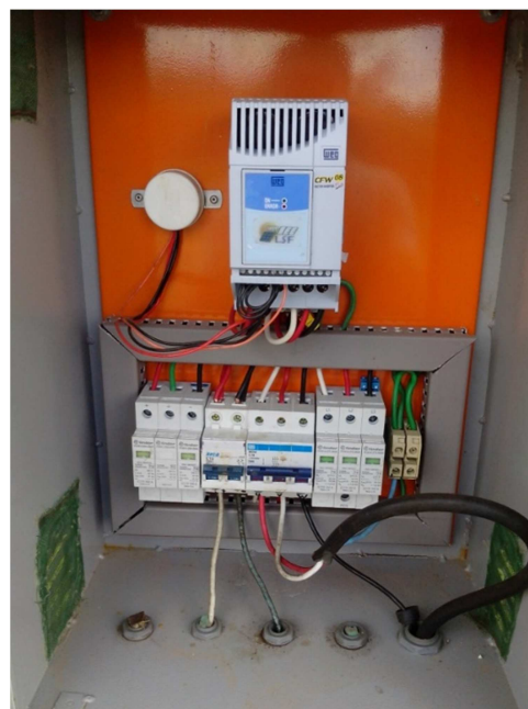
Figura 7: Quadro elétrico contendo o conversor de frequência e dispositivos de proteção.
