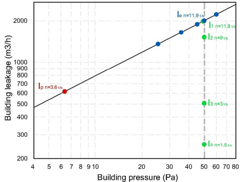
Figura 4: Curva de infiltración de la vivienda. Puntos azules: mediciones obtenidas, a 50 Pa equivalente a 11.9 Vol/h. Punto rojo: infiltración de la vivienda en m³/h a 6.35 Pa, presión de viento promedio para la localidad. Puntos verdes: I1= Vivienda en Albañilería de Ladrillo chilena, I2= Vivienda de hormigón, I3= Valor máximo de infiltración normado para una vivienda c/ventilación natural en Alemania y Austria, I4= Valor máximo de infiltración normado para una vivienda c/ventilación mecánica en Alemania y Austria.
