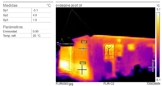
Figura 7: Imagen termográfica cara Sur.
