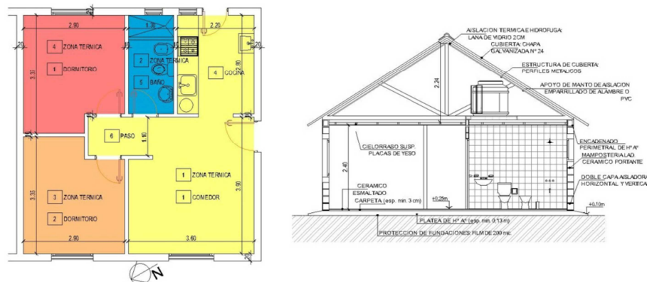
Figura 2: Planta de arquitectura de la vivienda junto con corte crítico.
