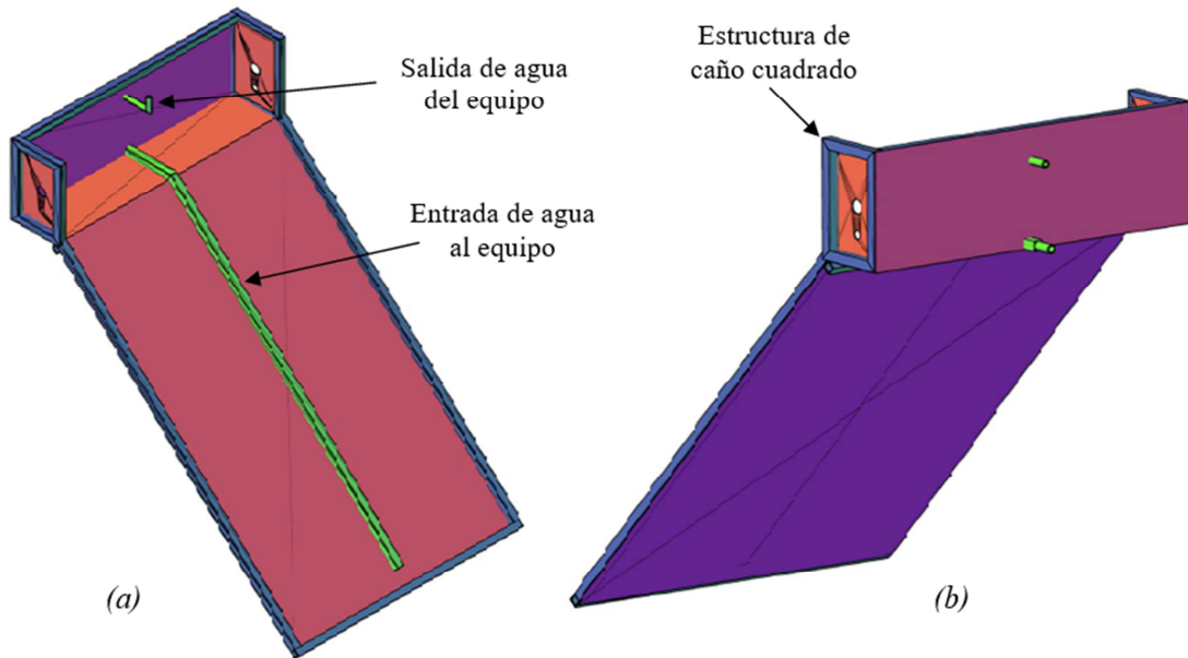
Figura 2: (a) Parte posterior del absorbedor-accumulador sin la chapa superior, vista de frente, incluyendo caños de entrada y salida; (b) parte posterior del absorbedor-accumulador sin la chapa superior vista de atrás.
